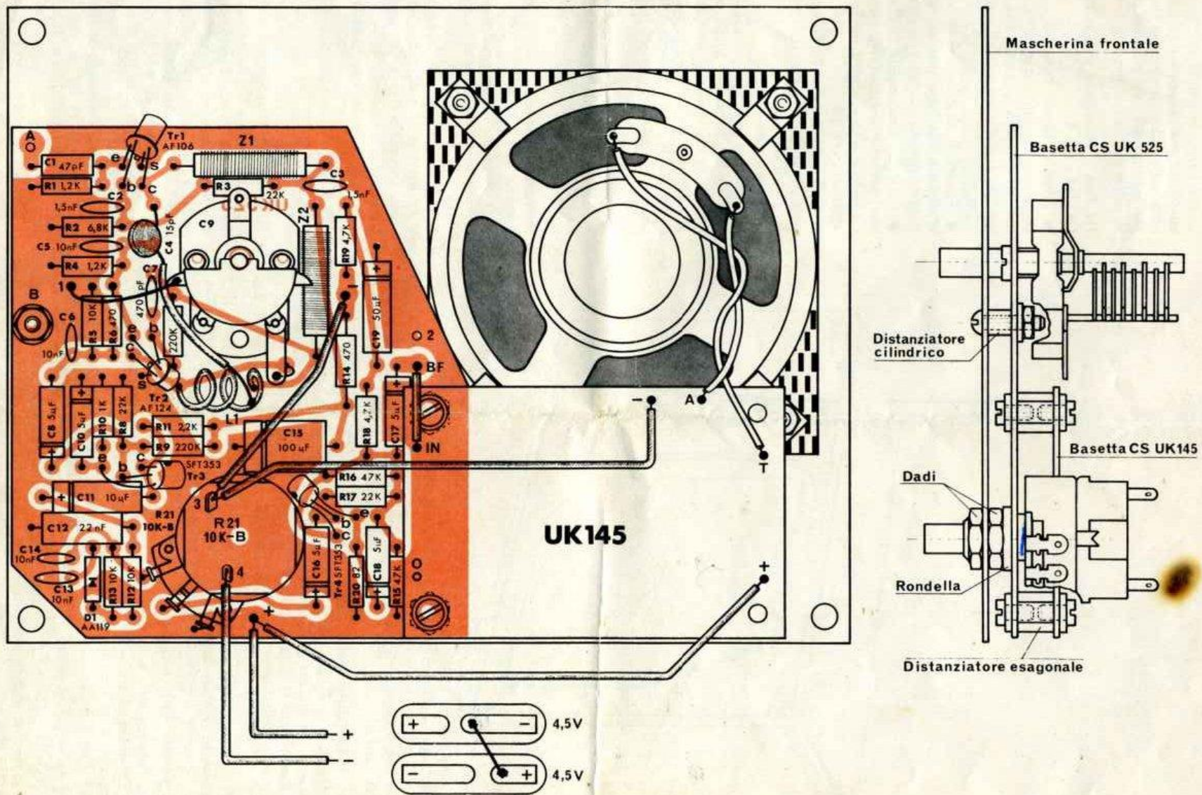
Fig. 5 - Montaggio dell'amplificatore UK 145 sul pannello recante i componenti del sintonizzatore UK 525/C.
